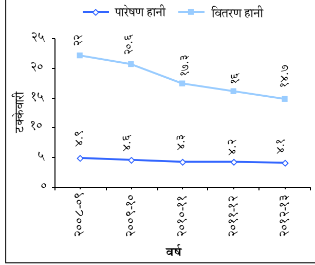
आलेख ९.५ : पारेषण व वितरण हानी
